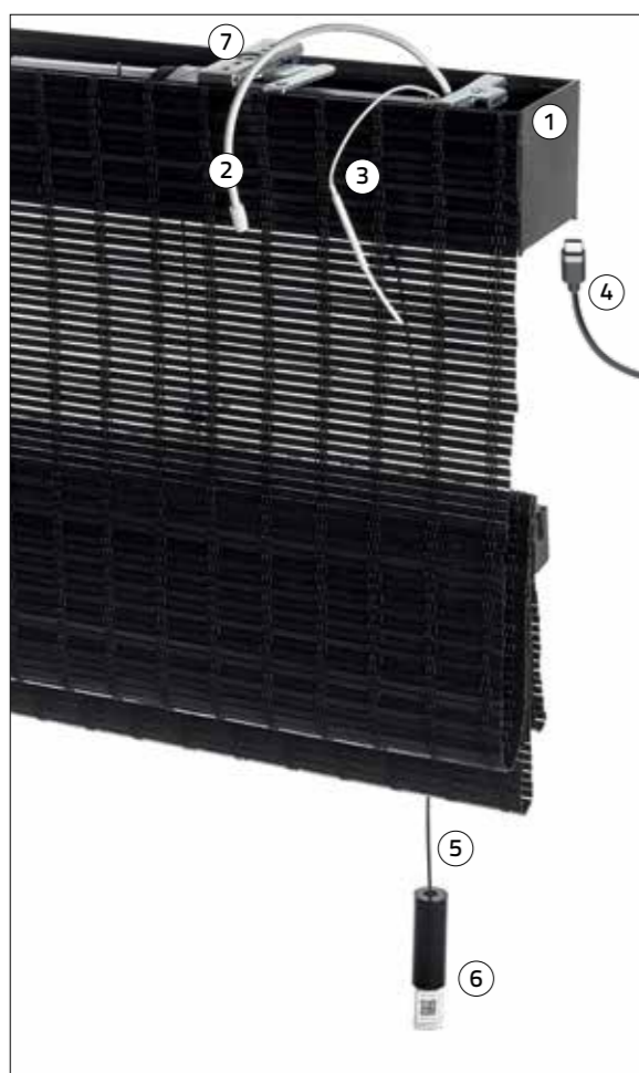
Vouwgordijn met CM-06 / CM-06-E-R batterijmotor
