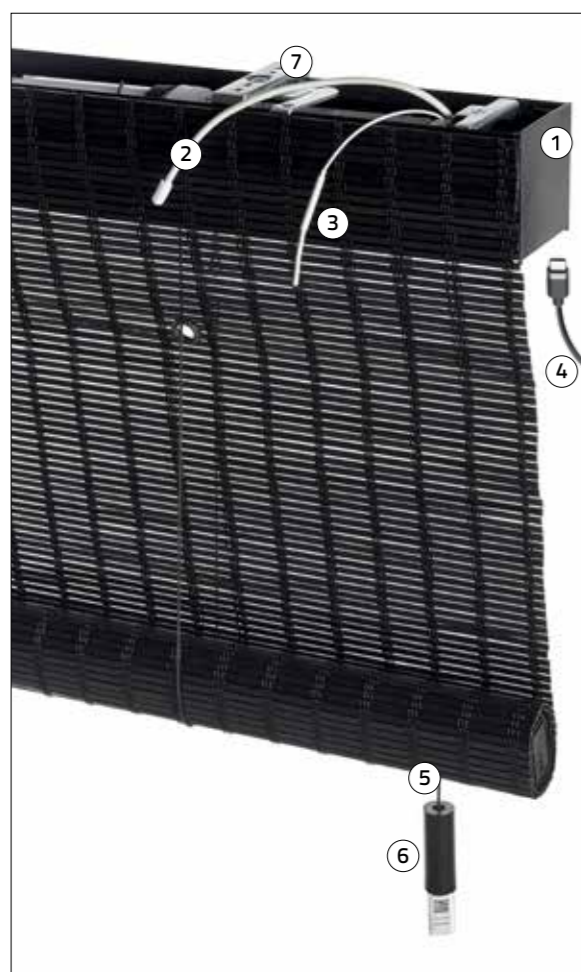
Roll Up met CM-06 / CM-06-E-R batterijmotor
